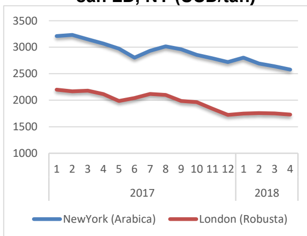
Hình 2: Biểu đồ biến động giá trên 2 sàn LB, NY (USD/tấn)
